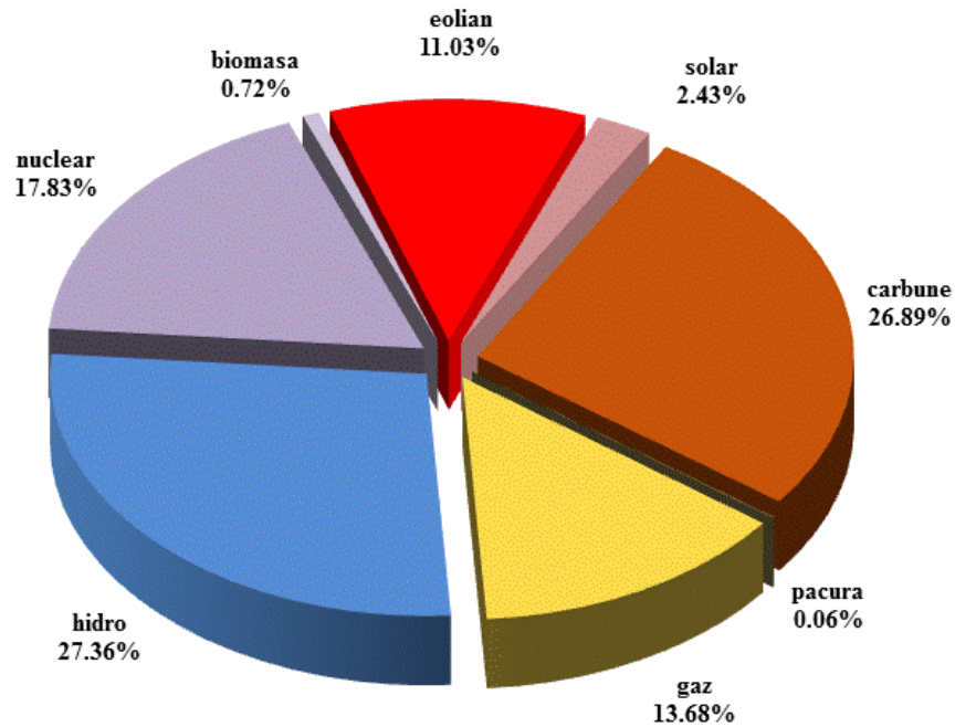
Structura pe tipuri de resurse a energiei electrice livrate în rețele de producători dispencerizabili și nedispencerizabili - 2015 -
